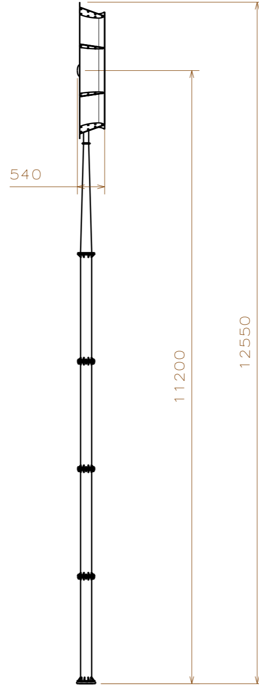
Left view Scale: 1:75
